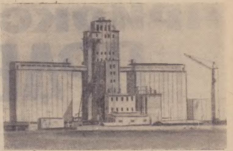
В селе Половинное Курганской области закончено строительство первой очереди крупнейшего в Зауралье элеватора (на снимке). Его силосные башни смонтированы из сборного железобетона. Весь процесс приемки, переработки и отгрузки зерна — автоматизирован.
